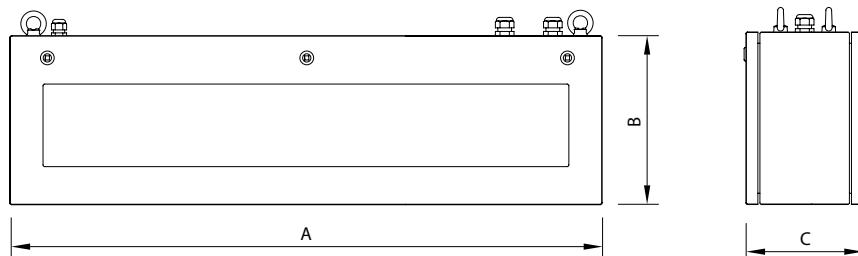
Visualizador doble cara
